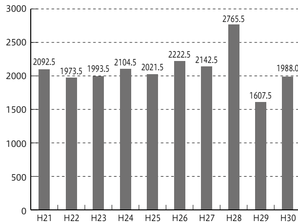
年間降水量の推移
