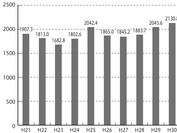
年間日照時間の推移
