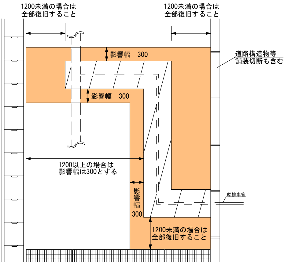
復旧平面図（標準）
