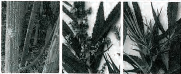
茎 雄花 雌花
