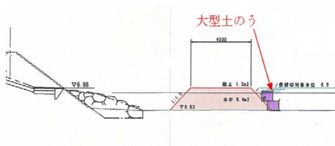
標準断面図
